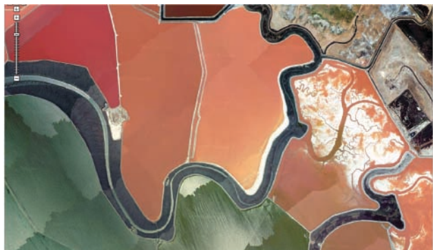
Кристализация
